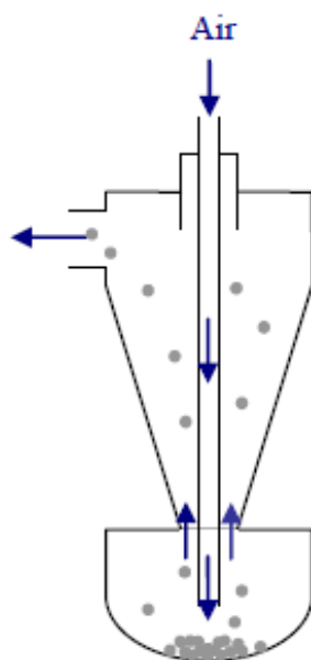
Schéma de fonctionnement du générateur
